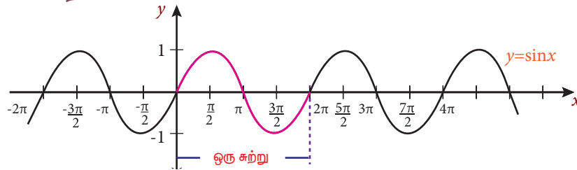
படம் 3.13 : y = \sin x
