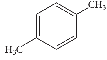
p-சைலீன் 1,4-டைமெத்தில் பென்சீன்
