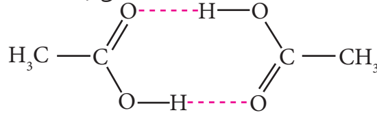
படம் 9.9 அசிட்டிக் அமிலம் (இருபடி)
