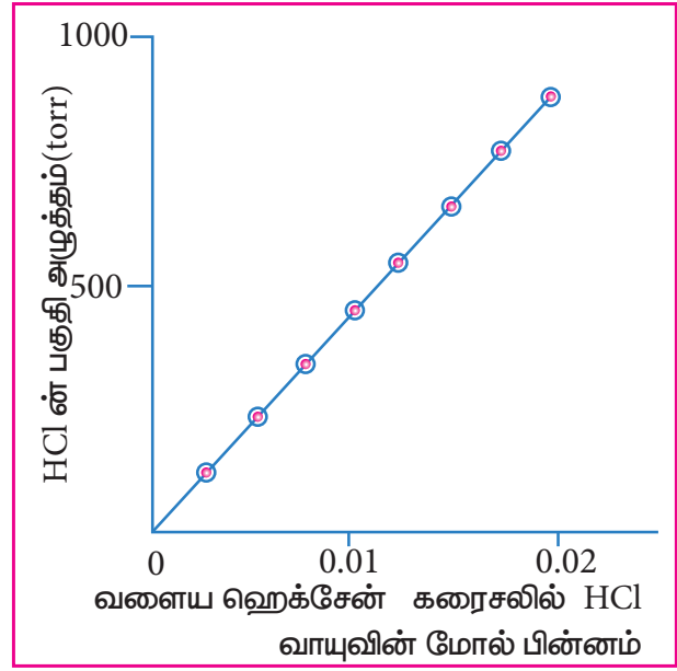
படம் 9.3 293K ல் வளையஹெக்சேனில் கரைந்துள்ள HCl வாயுவின் கரைதிறன்
