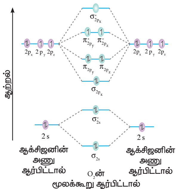
படம் 10.35. ஆக்சிஜன் (O 2 ) மூலக்கூறு ஆர்பிட்டால் வரைபடம்
